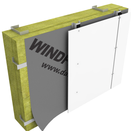
DAFA WindFoil 130 Plus som vindsperre i ventilert ytterveggskledning
