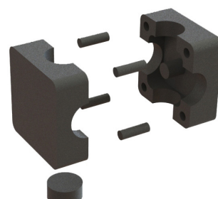
DAFAs egenproducerede radonbrønd som samlesæt.
